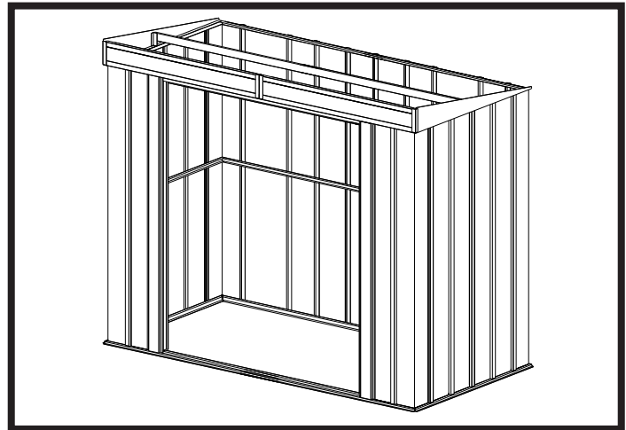
Türsturz, Giebel und Dachträger montieren
