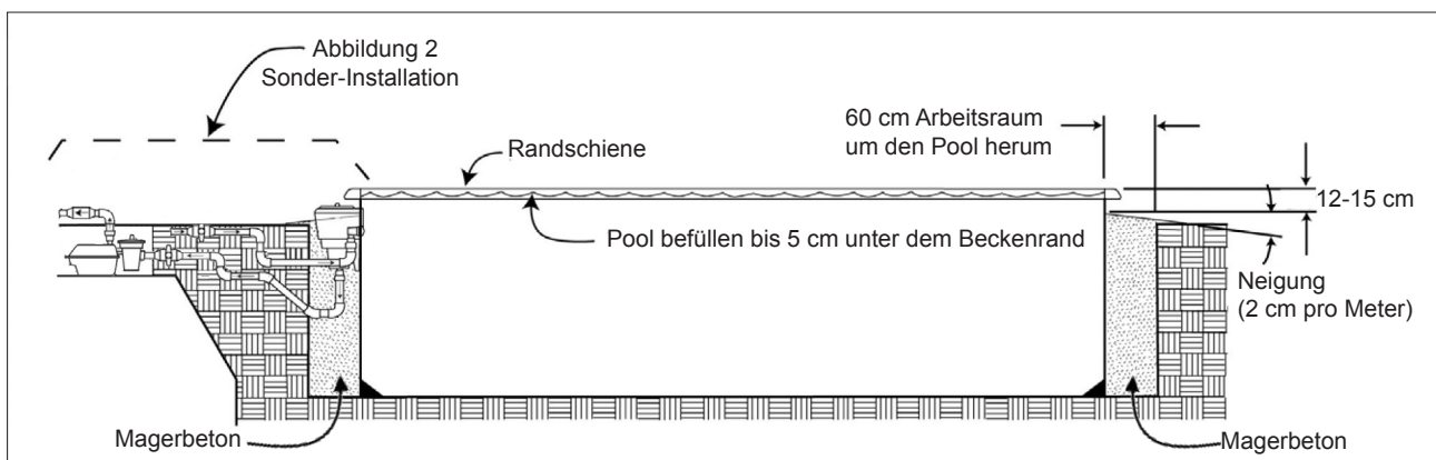
ABB. 1 - BAUMAßNAHMEN, WENN EIN POOL EINGRABEN WIRD
