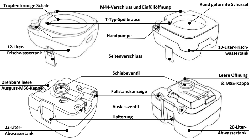
Abwassertank der Serien T und PT
